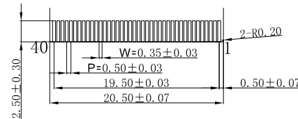
Detail:B Scale:4:1
