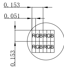
Detail:A Scale:40:1
