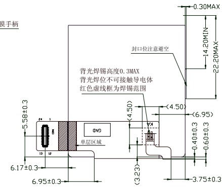
LCD-FPC弯折参考图
